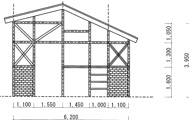
側面図
