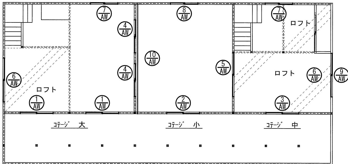
平面図
