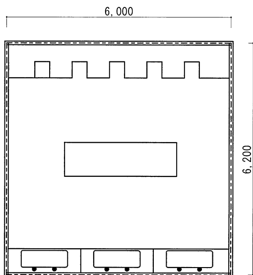
平面図
