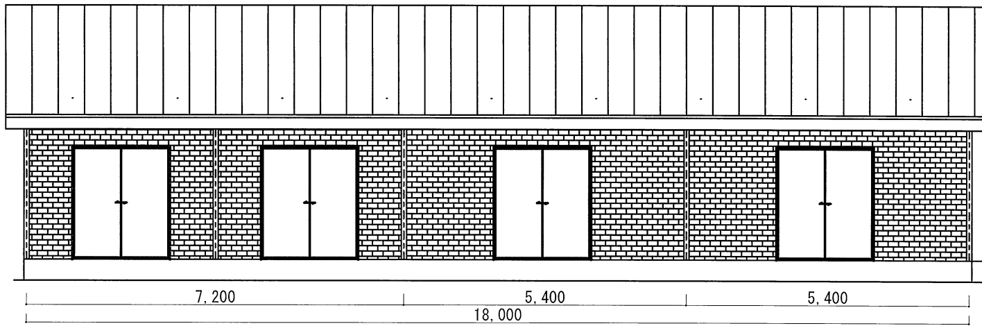
正面図
