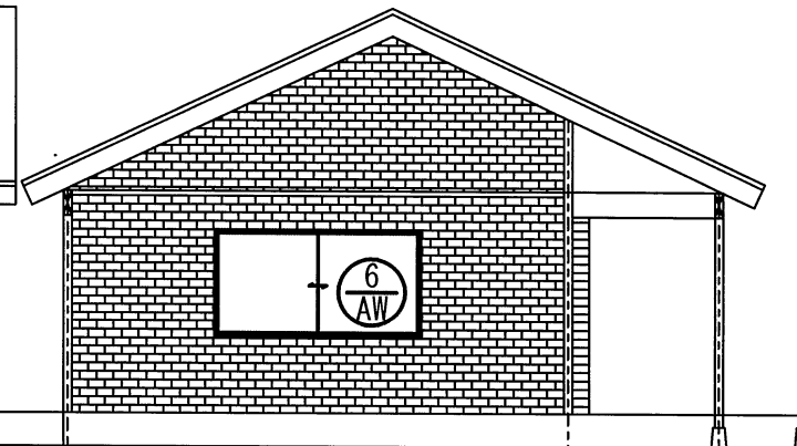
側面図
