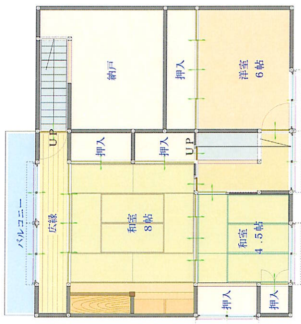
2階 平面図
