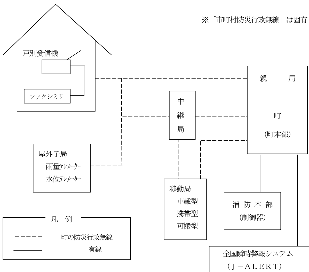
【 町 防 災 行 政 無 線 系 統 図 】
